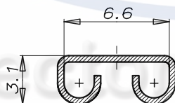
Section A-B
