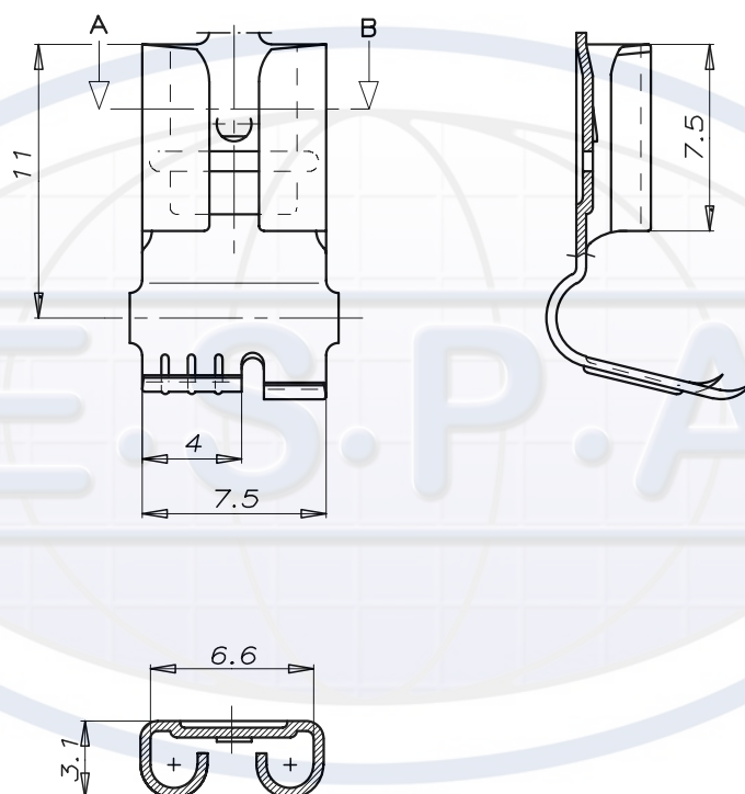
Section A-B
